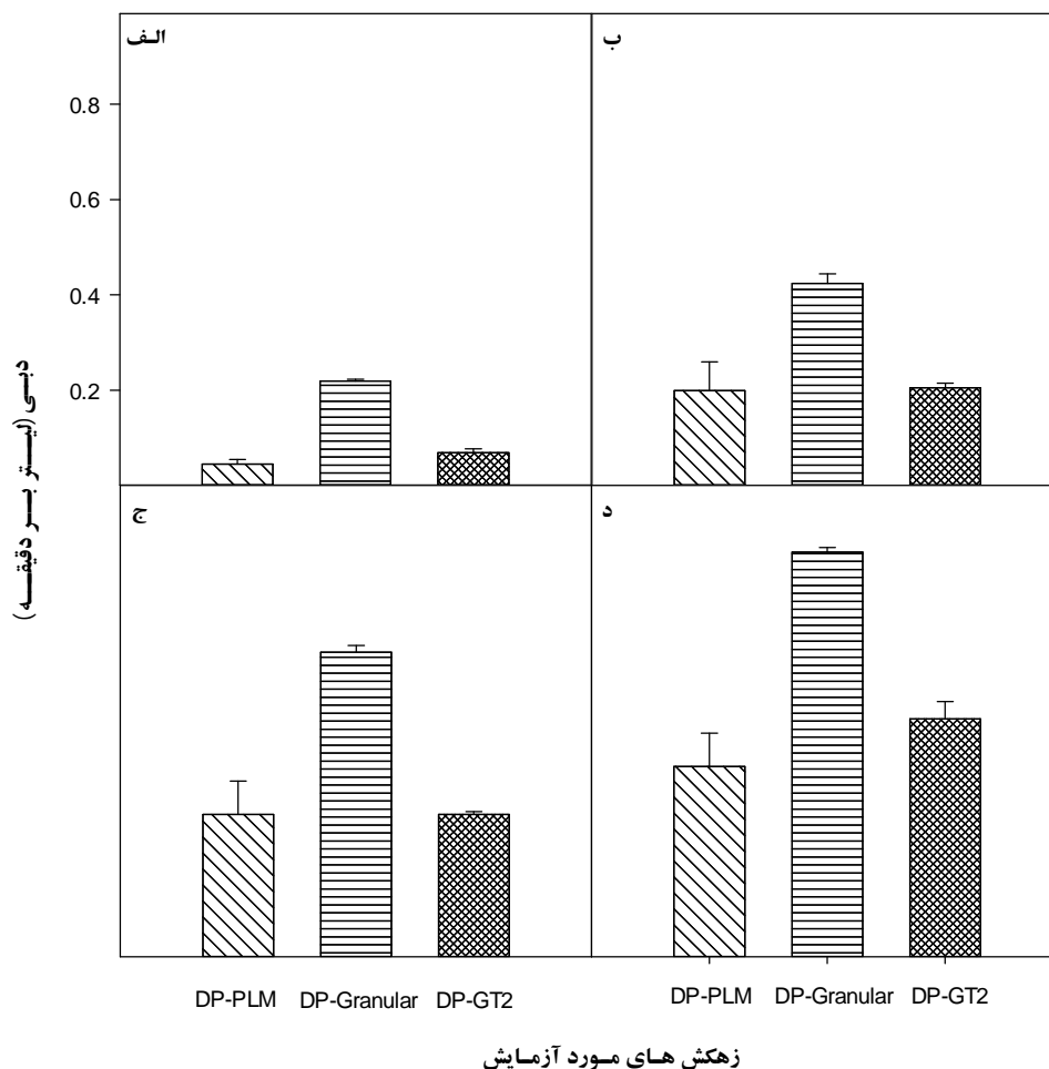
شکل (3): مقایسه دبی خروجی از زهکش برای زهکش های DP-PLM، DP-Granular و DP-GT2 در بارهای آبی الف - 45 سانتی متر، ب - 70 سانتی متر، ج - 90 سانتی متر و د - 110 سانتی متر
