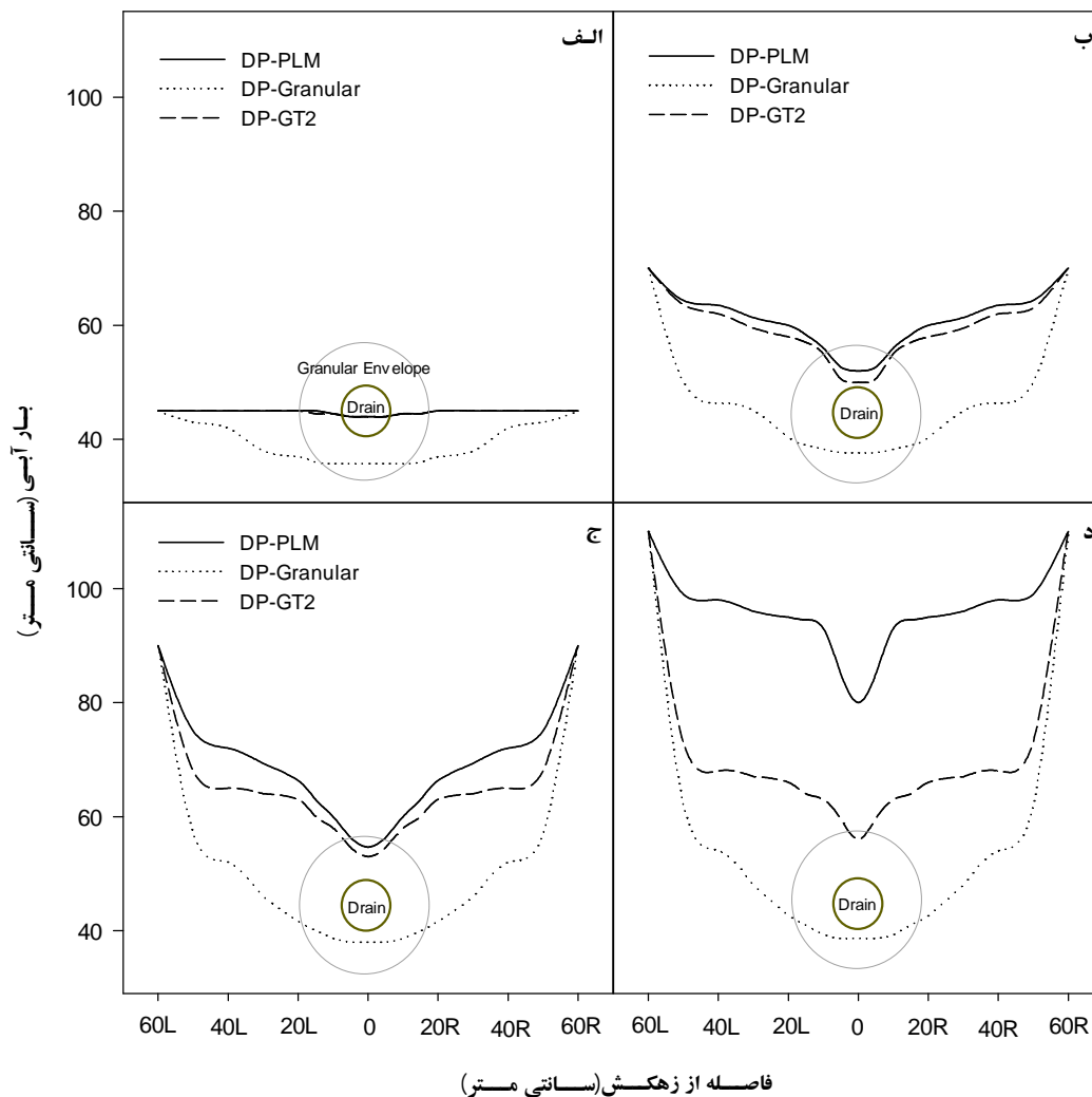
شکل (2): مقایسه وضعیت سطح ایستایی برای زهکش‌های DP-PLM، DP-Granular و DP-GT2 در بارهای آبی الف- 45 سانتی‌متر، ب- 70 سانتی‌متر، ج- 90 سانتی‌متر و د- 110 سانتی‌متر
